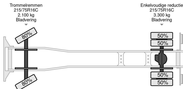
Mercedes-Benz 609 DK CREWCAB 4x2 3-WAY MEILLER KI...
